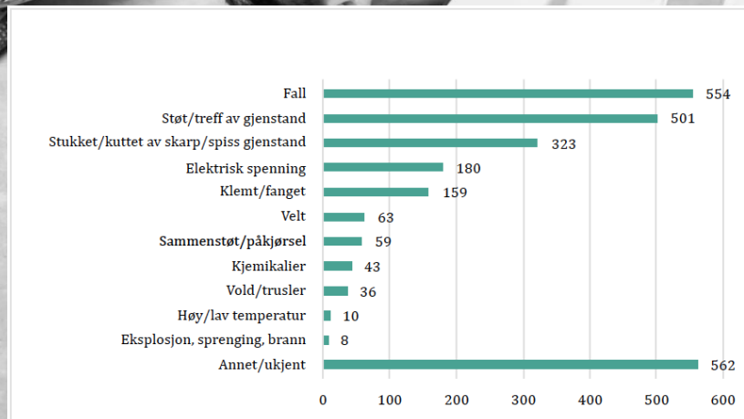
Figur 9: Meldte arbeidsskader i bygge- og anleggsnæringen i 2020, fordelt på ulykkestype. Kilde: SSB, Statistikkbanken tabell 11343.
